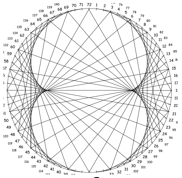
n → 3 n nefroida
